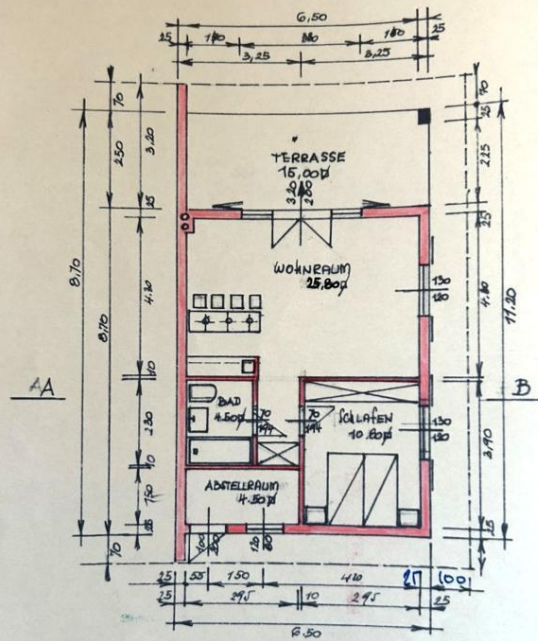
GRUNDRISS
