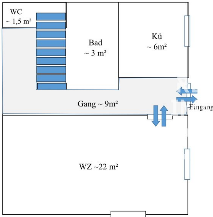
Erdgeschoss
