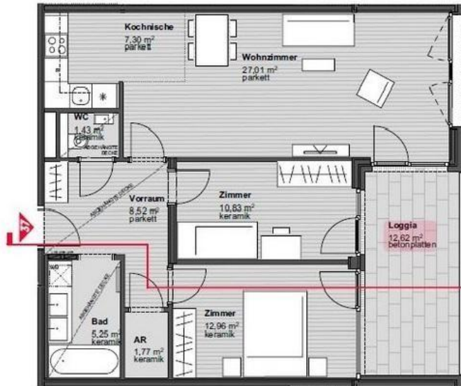
Grundriss | M 1:100
