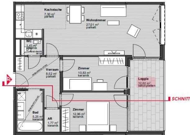
Grundriss | M 1:100
