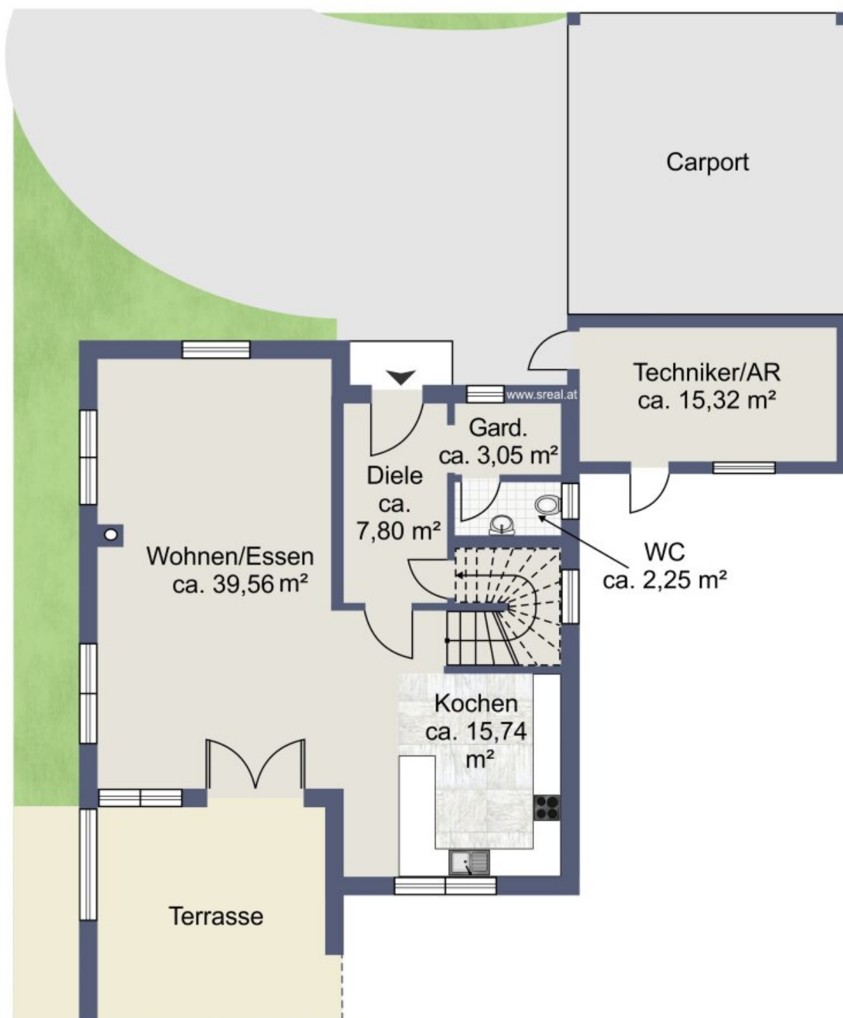
Skizze Erdgeschoss
