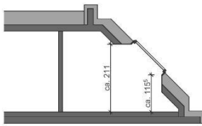
Systemschnitt A
