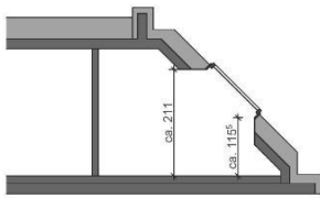
Systemschnitt A
