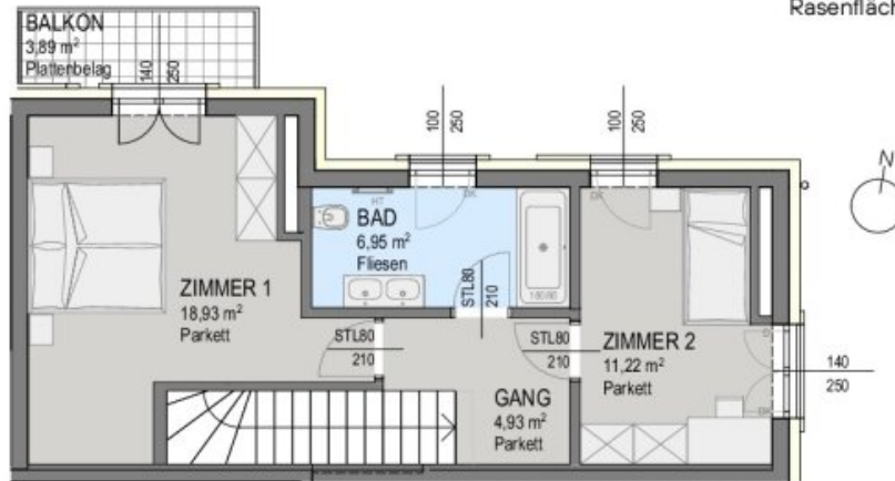
GRUNDRISS: ERDGESCHOSS
